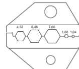
Crimpeinsatz profil
