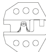
Crimpeinsatz profil
