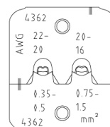
Crimpeinsatz profil
