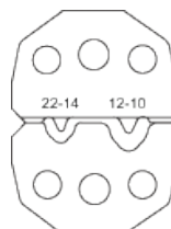
Perfil de matriz
