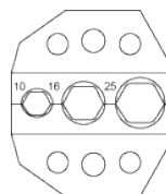
Profil de matrice
