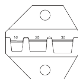
Profilo matrice
