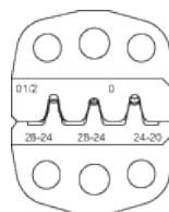
Profilo matrice
