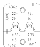
Profilo matrice
