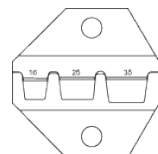
ダイの断面
