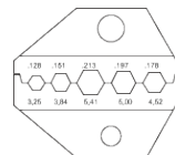
ダイの断面
