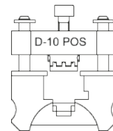
ダイの断面
