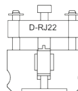
ダイの断面
