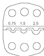
ダイの断面
