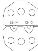
ダイの断面
