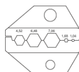
ダイの断面
