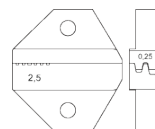
ダイの断面
