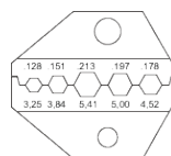
ダイの断面
