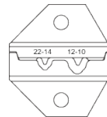
ダイの断面
