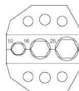
ダイの断面
