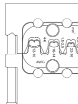
ダイの断面
