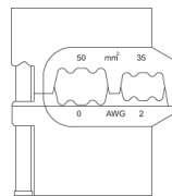
ダイの断面
