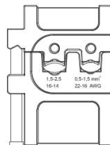
ダイの断面
