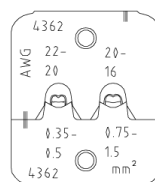
ダイの断面
